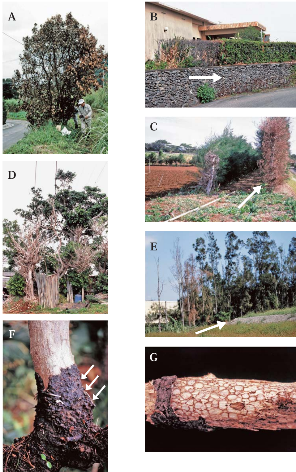
図ー 1 各種樹木に発生した南根腐病
