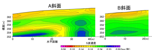
図－3 S波速度分布（桜島地区斜面）
