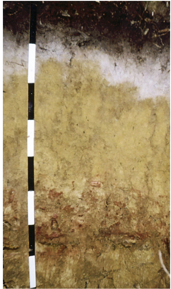
写真-1 表層グライ系赤黄色土の土壌断面
