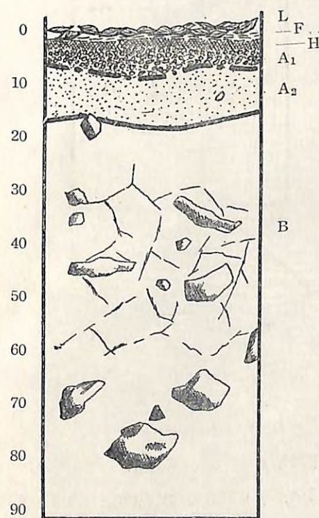
Fig. 4. Prof. No. 29. BB-soil.
