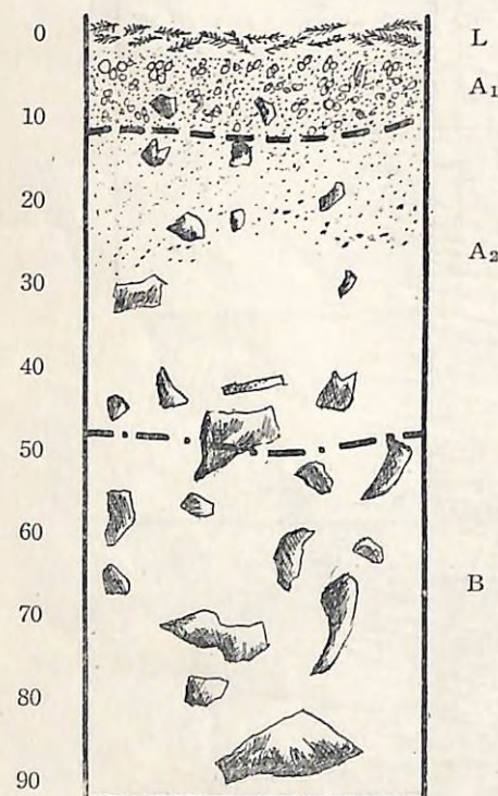
Fig. 14. Prof. No. 34. BD-soil.
