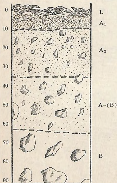
Fig. 11. Prof. No. 14. BD-soil.
