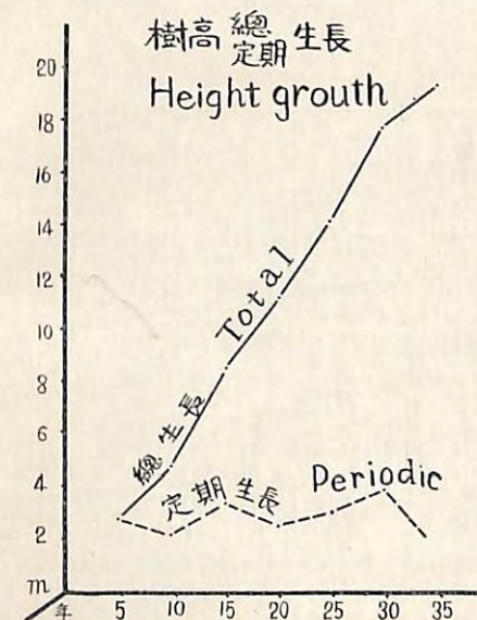
Fig. 35 Bd 型土壤に於けるスギの生長曲線 Growth curve of Cryptomeria japonica on Bd-soil.
