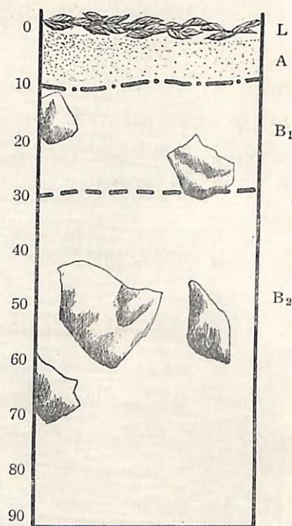
Fig. 13. Prof. No. 24. BD-soil.
