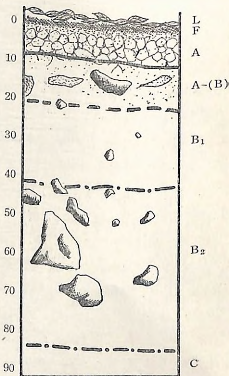
Fig. 8. Prof. No. 28. B 0 -soil.
