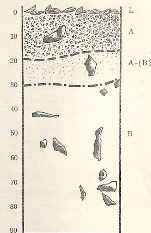
Fig. 16. Prof. No. 20. BE-soil.
