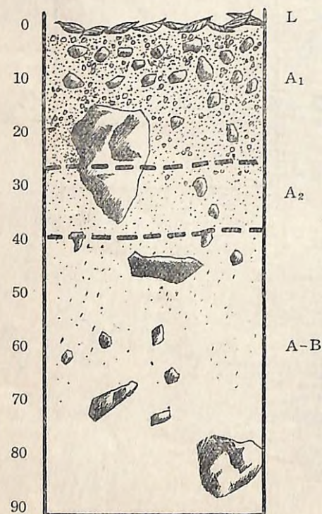
Fig. 17. Prof. No. 21. BE-soil.
