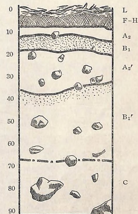
Fig. 18. Prof. No. 41. P DI -soil.
