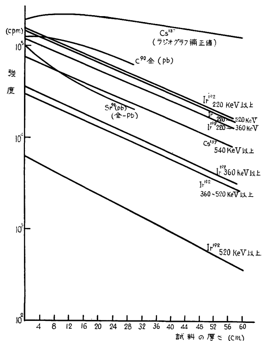
第17図 各波高領域計数値
