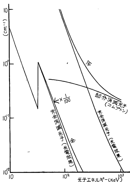
第2図 NaI (Tl) の断面積 (反応確率)
