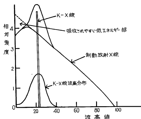
第4図 β 励起X線の波高分布 (模型)
