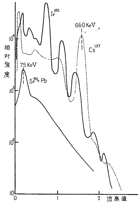
第 11 図 各線源の標準分布
