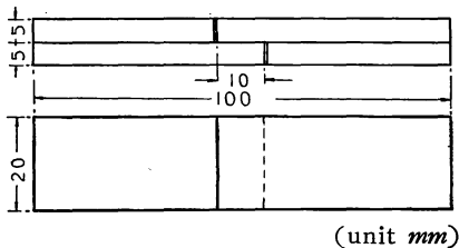
Fig. 1 試験片の形状
