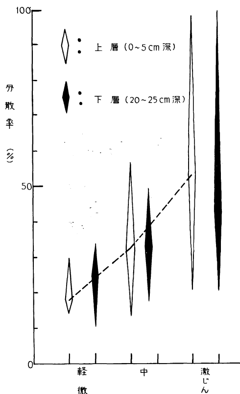
第8図 被災6か月後の場所からとった 土壌の分散率
