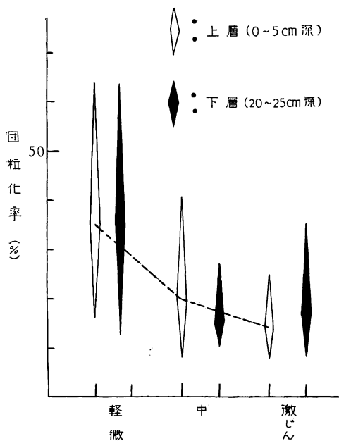
第 6 図 被災 6 か月後の場所からとった土壌の団粒量
