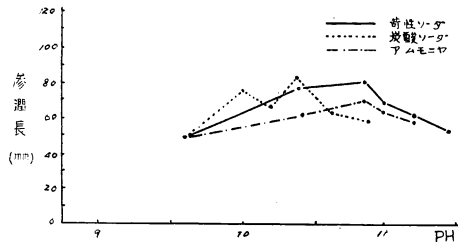
第5図(A) pH と滲潤長の関係 試験材: 2.5 \times 5 \times 60 cm Na-PCP: 1% 溶液 処理条件: 前排气 700mm 20min, 圧力 3.5 \text{ kg/cm}^2 , 加圧時間 30min, 温度 25^\circ\text{C}
