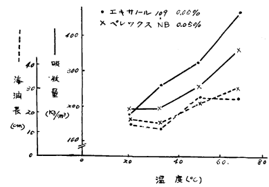
第6図 活性剤添加による温度と滲潤長, 吸収量の関係 Na-PCP: 1% 溶液 処理条件: 前排气 650mm 20min, 圧力 7 \text{ kg/cm}^2 , 加圧時間 120min
