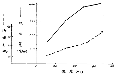
第 3 図 温度と滲潤長, 吸収量の関係 Na-PCP: 1% 溶液 処理条件: 前排気 650mm 20min, 圧力 7kg/cm², 加圧時間 120min
