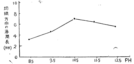
第5図(B) pH と滲潤長との関係 試験材: 5 \times 5 \times 6 cm Na-PCP: 1% 溶液 処理条件: 前排气 700mm 10min, 圧力 3.5 \text{ kg/cm}^2 , 加圧時間 20min, 温度 25^\circ\text{C} pH 補正剤: 苛性ソーダ
