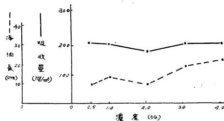
第 4 図 濃度と滲潤長, 吸収量の関係 処理条件: 前排気 650mm 20min, 圧力 7kg/cm², 加圧時間 120min, 温度 20°C
