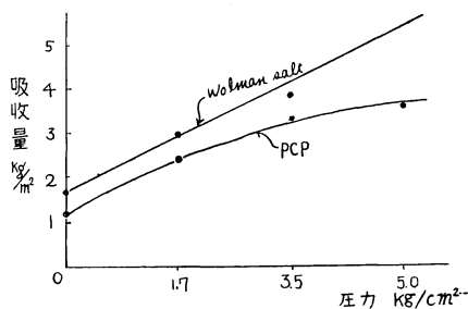
第8図 圧力と吸収量の関係
