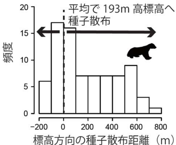
図1：（左上）結実木から採取した種子の酸素安定同位体比と標高の関係。標高が高いほど同位体比が減少しています。この関係を利用することで散布された種子の親木の標高が求まるため、標高方向の種子散布が評価できます。（右上）ツキノワグマによる標高方向への種子散布の頻度分布。標高の高い方に偏って種子が散布されています。（左下）テンによる種子散布の頻度分布。ツキノワグマより平均の散布距離が短いことがわかります。（右下）哺乳類による種子散布の模式図。山麓から山頂にかけて植物の開葉や結実が進み、それを哺乳類が追いかけた結果、種子が標高の高い方に偏って散布されたと考えられます。
