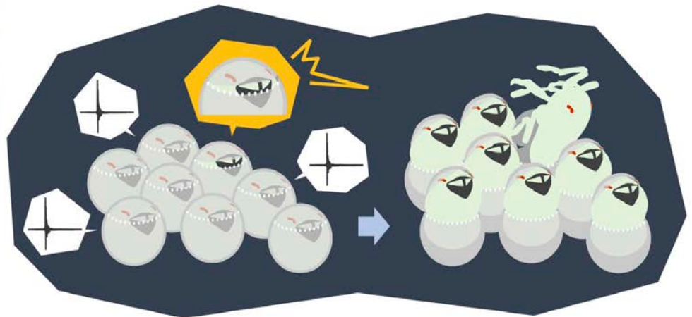
図. クサギカメムシの卵塊では、一つの卵が孵化を始めて殻が割れた振動を合図に一斉に孵化が起こる。
