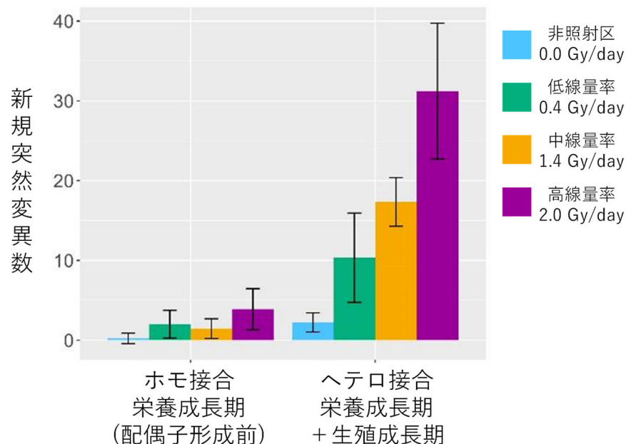
図 2. 検出された突然変異部位におけるホモ接合とヘテロ接合の数. ホモ接合とヘテロ接合の割合から、突然変異発生時期の全体的な傾向について推測できる。
