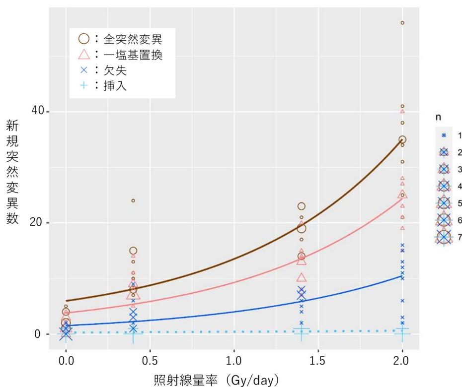
図 1. 照射したガンマ線線量と観察された突然変異数. 茶色は全ての突然変異、桃色は一塩基置換、青色は欠失、水色は挿入変異の突然変異数を示す。回帰曲線は統計モデリングによる予測値を示す。
