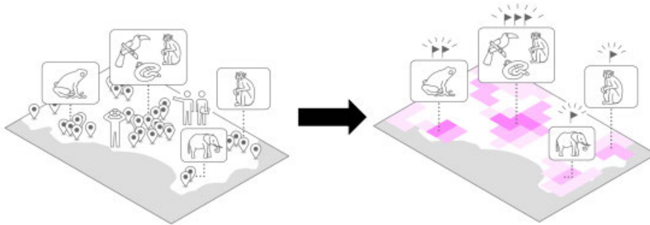
図 1: GBIF のデータから 7143 種の生物種のデータをもとに、「保全優先度」(CP、0~1)を 0.5^{\circ} グリッド (約 60km 四方) ごとに計算した。濃いピンクほどその場所の生物種が失われることによる生物多様性の損失が大きく、無色はほとんど生物が生息していない様子を表している。
