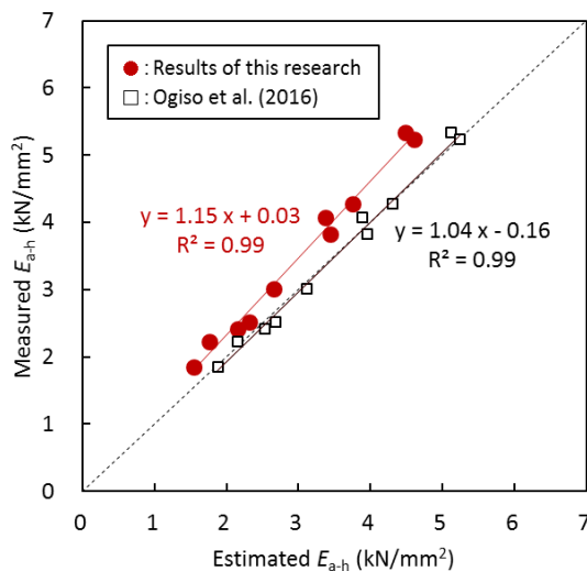
Fig. 9. CLT の面内曲げ試験における見かけのヤング係数 ( E_{a-h} ) および曲げ強さ ( \sigma_{b-h} ) の推定値と実測値の比較 Comparison between the estimated and measured E_{a-h} and \sigma_{b-h}
