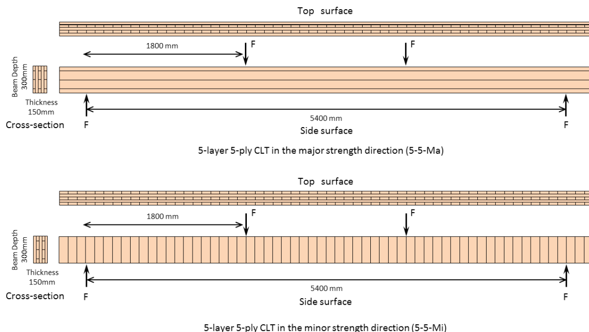
Fig. 2. CLT 試験体の面内曲げ試験（5層5プライの例）
