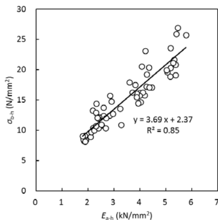
Fig. 5. CLT 試験体の見かけの曲げヤング係数 ( E_{a-h} ) と曲げ強さ ( \sigma_{b-h} ) の関係 Relationship between E_{a-h} and \sigma_{b-h} of CLT specimens
