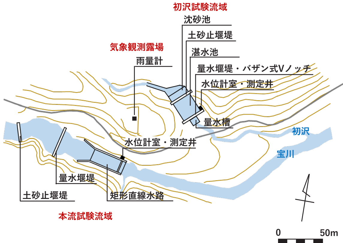
Fig. 2. 宝川森林理水試験地の観測施設
