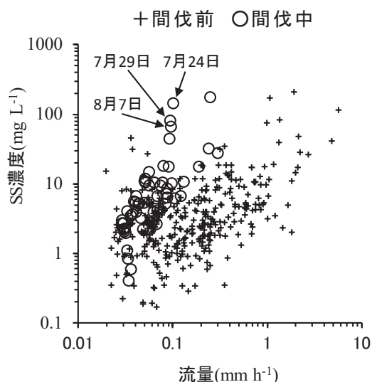
Fig. 5. 2013 年間伐における間伐前と間伐中の流量と SS 濃度との関係
