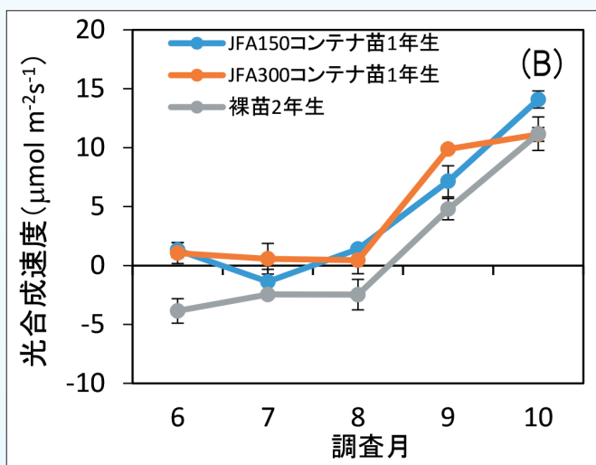
図1 カラムツのコンテナ苗（1年生）と裸苗（2年生）の比較
