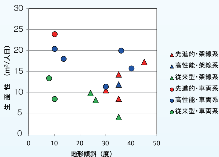
図1 伐出システムの生産性
