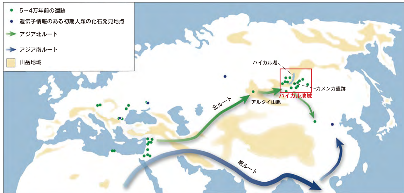
図1 氷期のアジアにおける人類の移動ルート 5～4万年前の氷期に起きたアフリカからアジアへの人類の移動は、バイカル地域を経由する北ルートと東南アジアを経由する南ルートがあったとされる。
