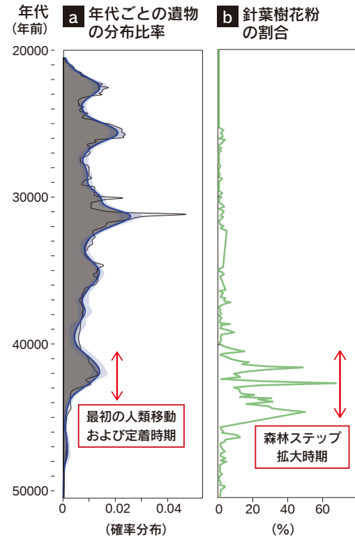
図2 バイカル地域から出土した遺物の年代ごとの分布比率とバイカル湖底の泥に含まれる針葉樹花粉の割合の変化 a 約4万4000～4万年前に最初のピークがみられ、最初の人類移動および定着が生じた。b 約4万5000～4万年前に針葉樹が多く、イネ科などを含んだ森林ステップが発達した。 (Shichi et al. 2023 を改変)
