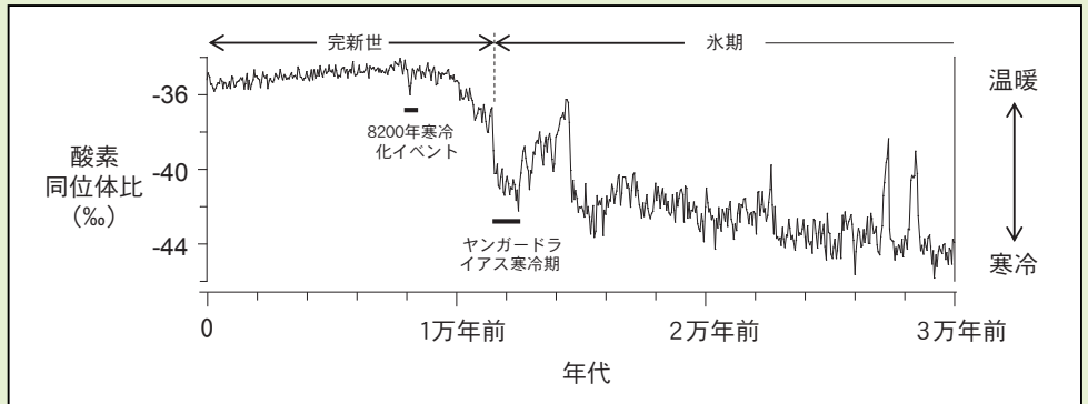
図1 グリーンランドにおける過去3万年間の気候変動 (North Greenland Ice Core Project members 2004より作成) 暖かくなると「軽い」酸素同位体 16 Oが先に蒸発し、相対的に「重い」酸素同位体 18 Oの割合が高くなることから、グリーンランド氷床中の 18 Oと 16 Oの比率の変化によって過去の気候を復元することができます。グリーンランドでは、ヤンガードライアス寒冷期には現在より15℃ほど、8200年寒冷化イベント時には3℃ほど気温が低下したとされます。
