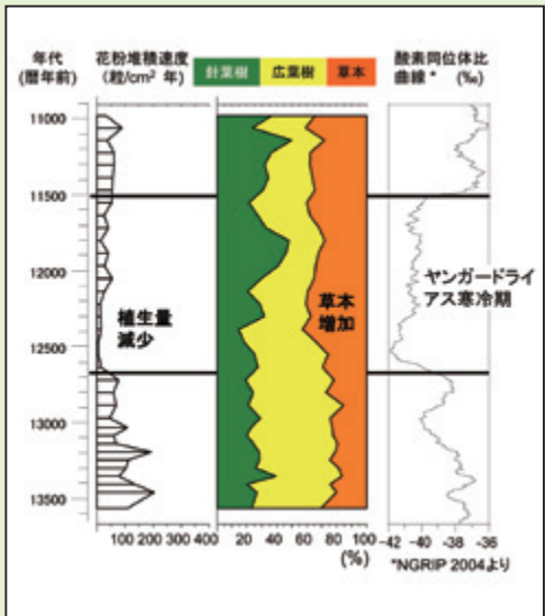
図2 ヤンガードライアス寒冷期における花粉産出割合の変化
