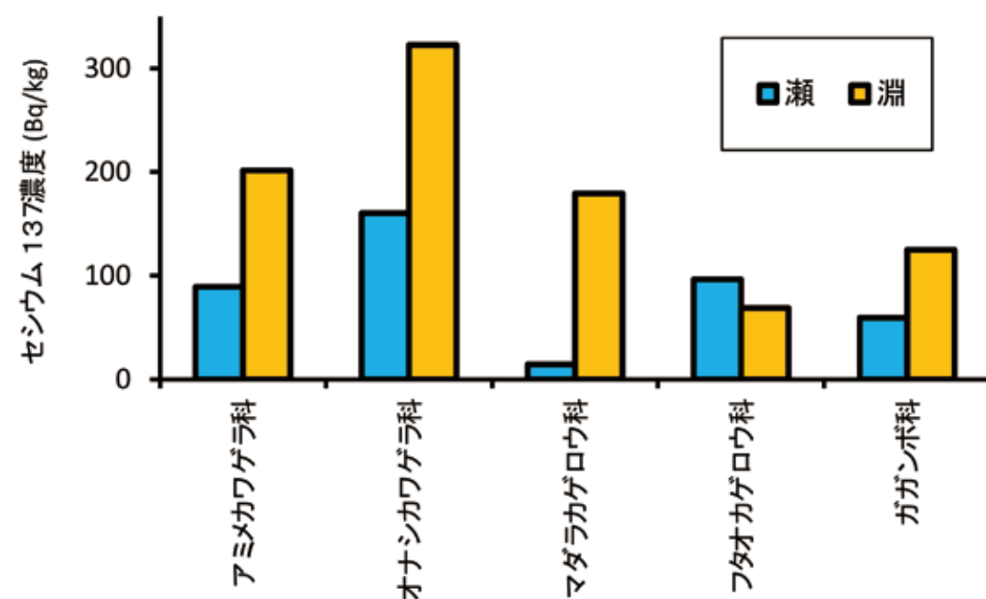
図2 瀬および淵に生息している5科の水生昆虫のセシウム137濃度
