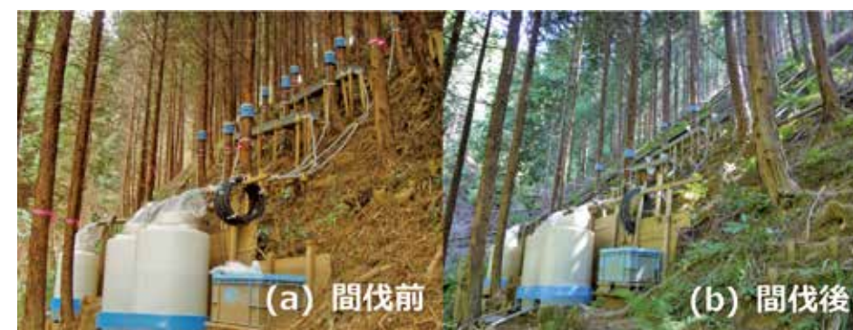
図2 (a) 間伐前、(b) 間伐後の遮断プロット内の様子。大型雨樋で樹冠通過雨、樹木周囲（間伐前10本、間伐後5本）に巻いたウレタンマットで樹幹流下雨を集め、大型タンクに導水して貯留量を測定した。
