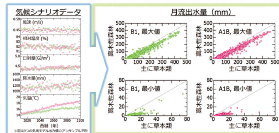
図2 温暖寡雨な山陽の森林小流域を対象に気候シナリオ別に推定された21世紀末までの月流出水量の最大値と最小値の植被状態による違い
