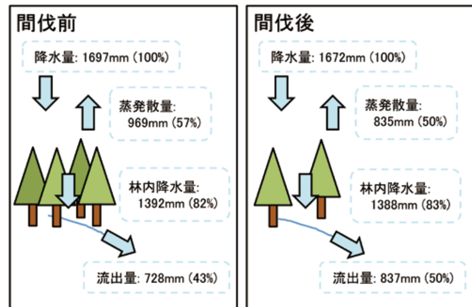
図3 間伐による水収支の変化。 間伐前後それぞれ3年間の平均値で示した。( ) 内は降水量に対する比率
