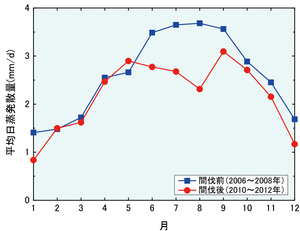
図4 間伐による蒸発散量の変化
