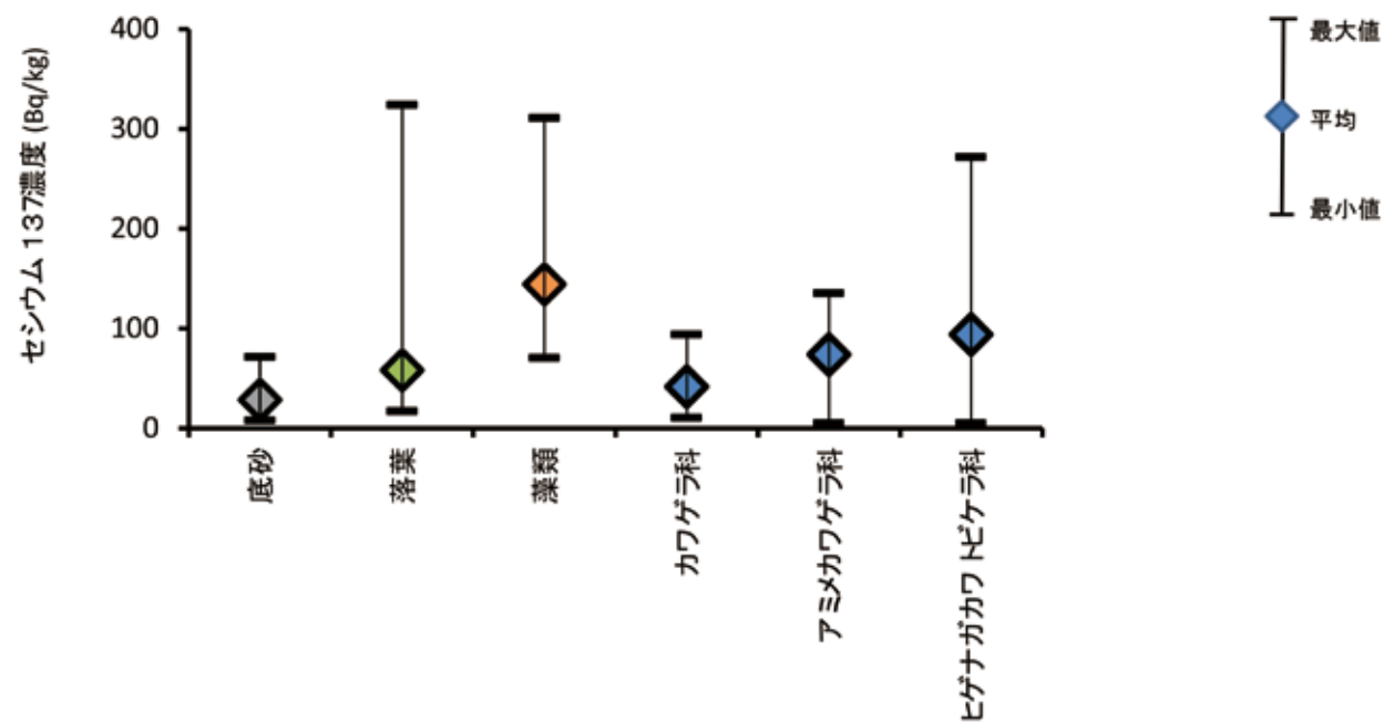
図1 中禅寺湖周辺河川における底砂・落葉・藻類・3科の水生昆虫のセシウム137濃度
