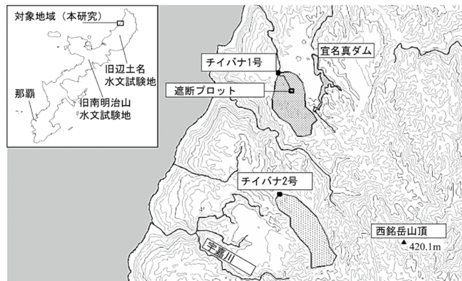
図1 研究対象地の位置
