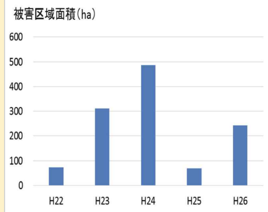
近年の凍害被害面積（全国） ※凍害はその年の気象条件により、被害の変動が大きい。
