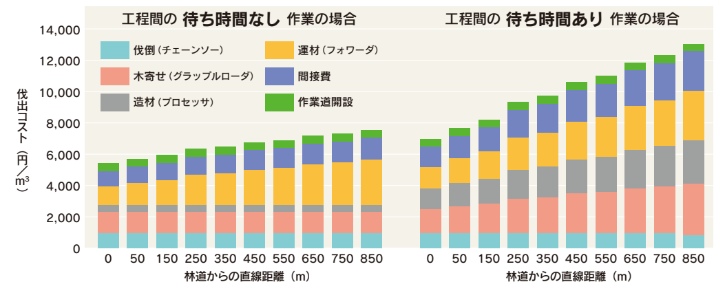
図2 林道からの直線距離に応じた伐出コスト カラマツ地位指数22の場合。「地位指数」とは、林齢と上層木の樹高から、その土地の生産力を示した指標値。 出典：宗岡寛子ら(2020)北の森だより 23:6-7
