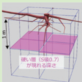
ケヤキ
