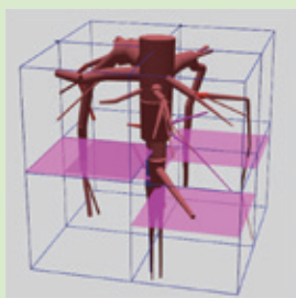
クロマツ
