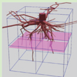
カシワ
