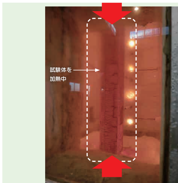
写真5 耐火試験
