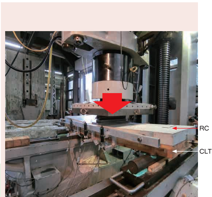
写真4 合成スラブ試験
