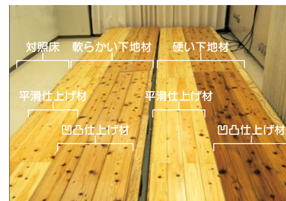
写真1 4種類のモデル床と対照床 奥行7.2mの4種類の床を作成して用いた。対照床は実験室の床(いちばん左側)を使った。
