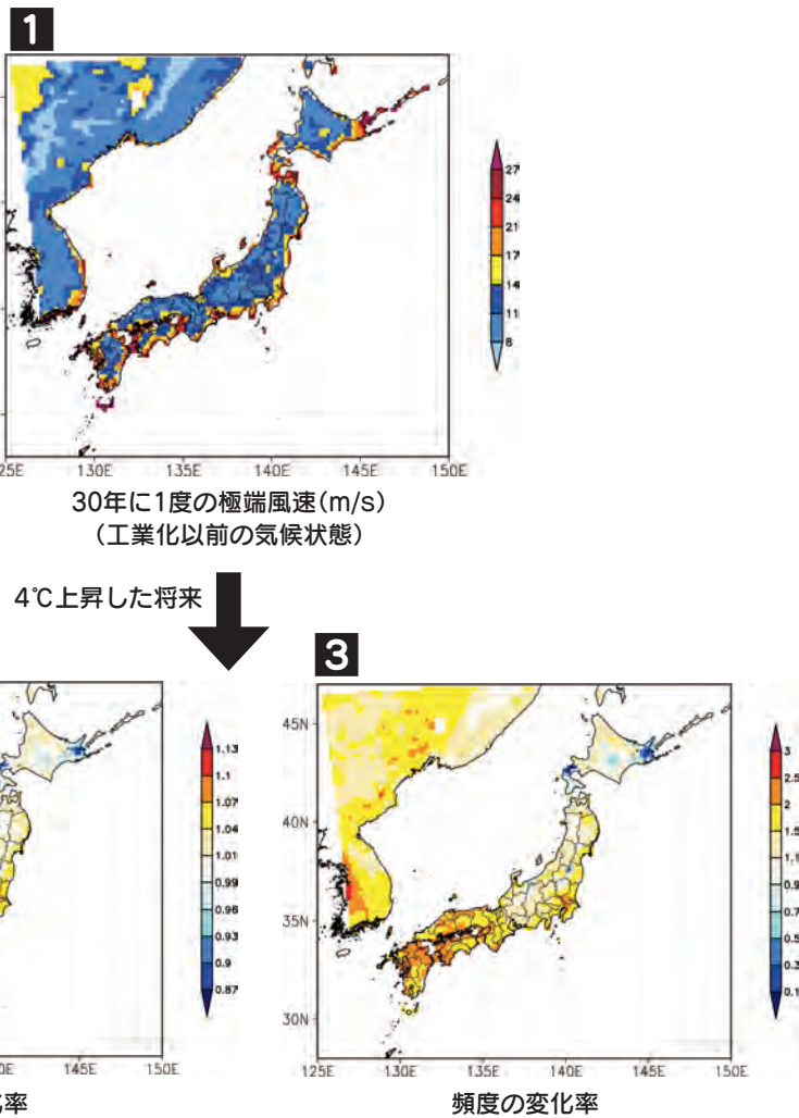
図2 30年に1度の極端風速の将来変化
