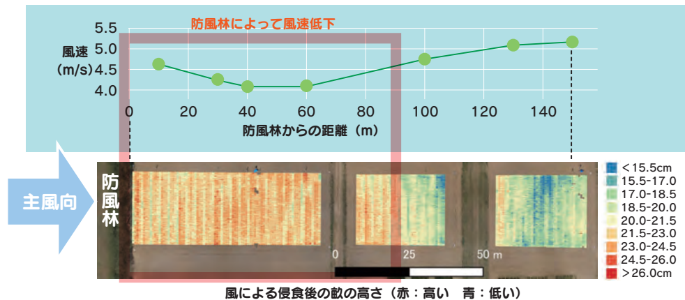
図2 防風林風下における風速とドローンから得られた畝の高さの分布 風速は、侵食が発生した日の平均。防風林によって風速が低下した場所では、強風後にも畝が高いまま維持されており、侵食されていなかった。(Iwasaki et al. (2024)の図を一部改変)
