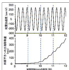
図2. 与えた地震加速度と崩壊初期の土塊移動量
