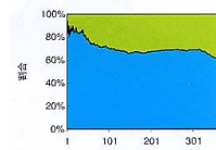
図4 南谷の森林消失による日流出量の増加割合
