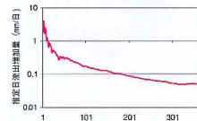
図3 南谷の森林消失による日流出量の増加量 (図2の赤線の値から緑線の値を引いた 値の19年分を平均したもの)
