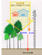
図1. 森林におけるエネルギー・水蒸気の交換
