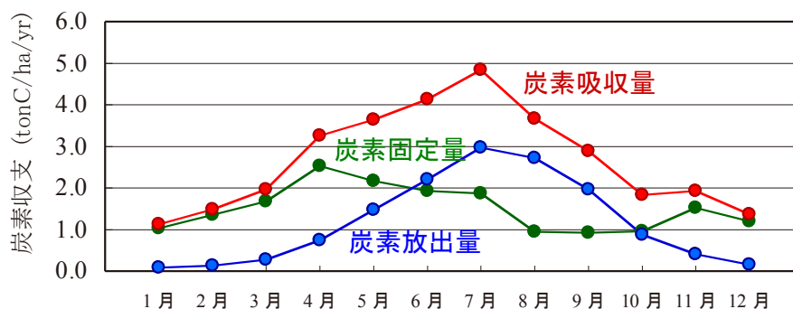
図4 スギ人工林における炭素収支の季節変化のシミュレーション
