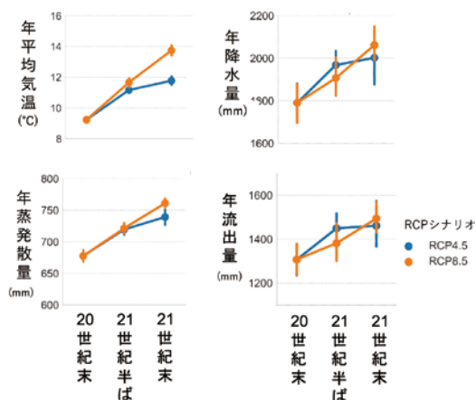
図2 日本の森林域における年平均気温、年降水量、年蒸発散量及び年流出量 いずれの値も時代と共に上昇している傾向が見られました。
