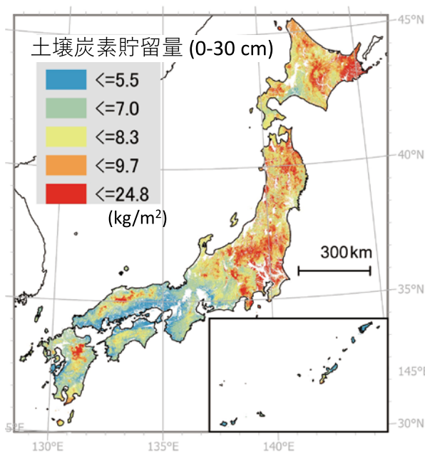
図3 全国の土壌炭素貯留量
