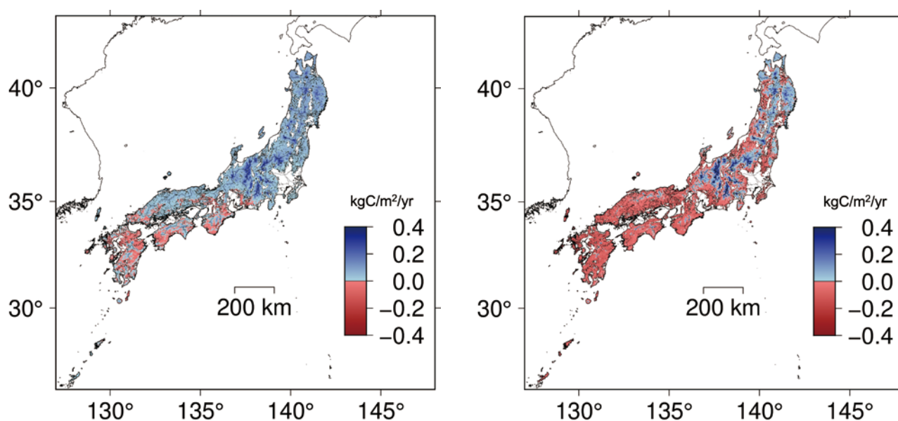
図1 CO 2 排出量が少ない（RCP2.6）シナリオの将来のスギ林の純一次生産量の変化 (将来(2096～2100年)－現在(1996～2000年))。青色が増加、赤色が減少。 (左) 世界の5つの研究機関が予測した気候モデルで進む場合の推定の平均値。 (右) 5つの中で気温上昇が最も大きいと予測された気候モデルのように進む場合。 計算結果は https://zenodo.org/record/5105060 からダウンロードできます。
