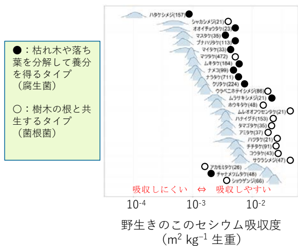
図3 野生きのこの放射性セシウムの吸収しやすい枯れ木や落ち葉を分解して生活するタイプのほうが樹木の根と共生して生活するタイプより放射性セシウムを吸収しにくい傾向にあります。
