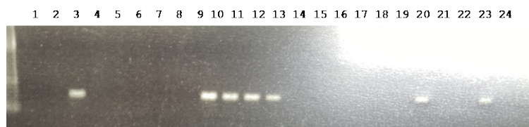
図3 高温発生型検出の選抜マーカーによる解析結果
