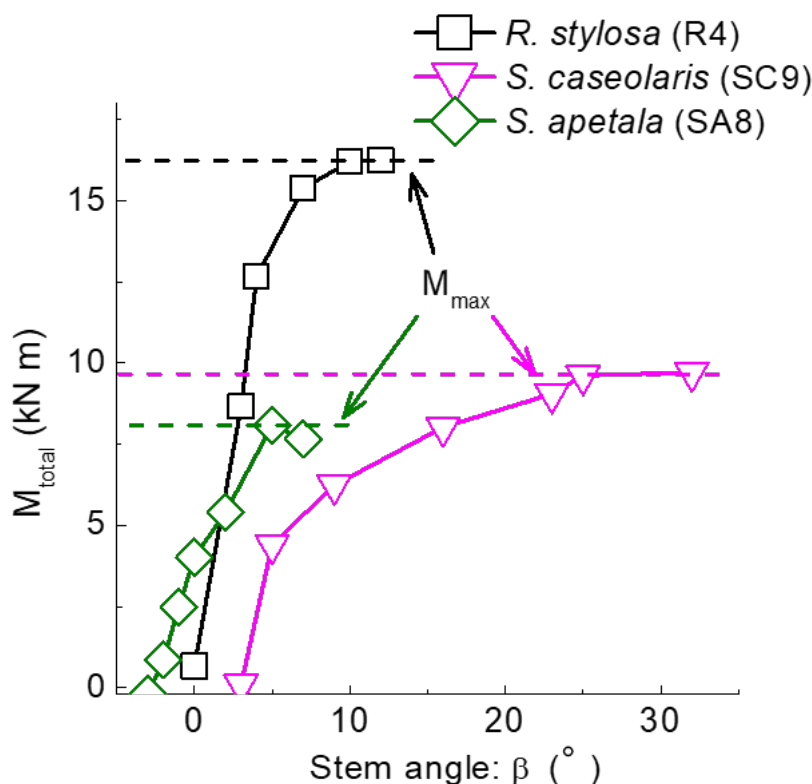
図 4-4-2-5 マングローブ引き倒し試験時における M_{total} と幹角度の関係
