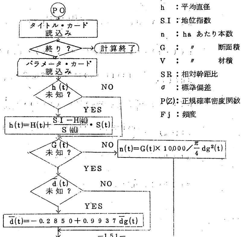
図-1 プログラムの計算手順のフロー・チャート
