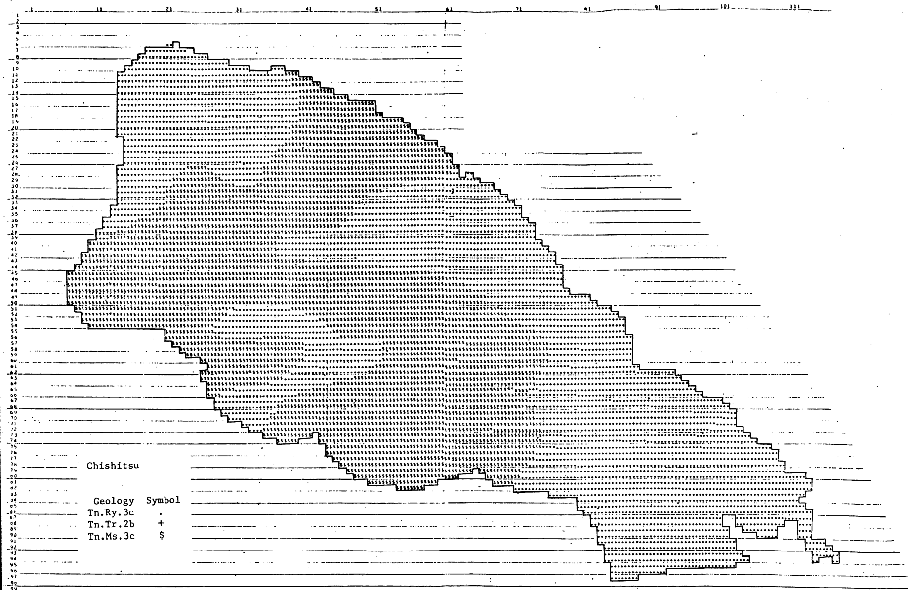
図6 表層地質図
