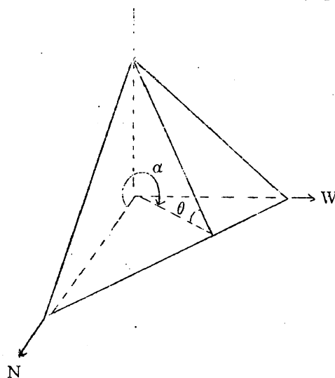
図-13 地形解析
