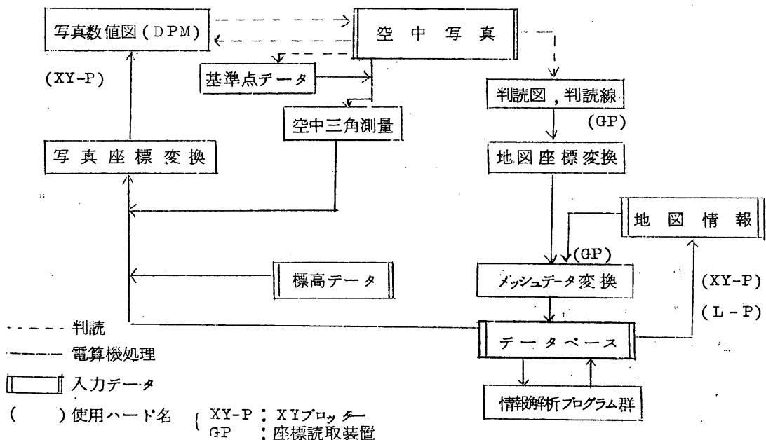
図-1 メッシュ方式データバンクへのデータ収集システム
