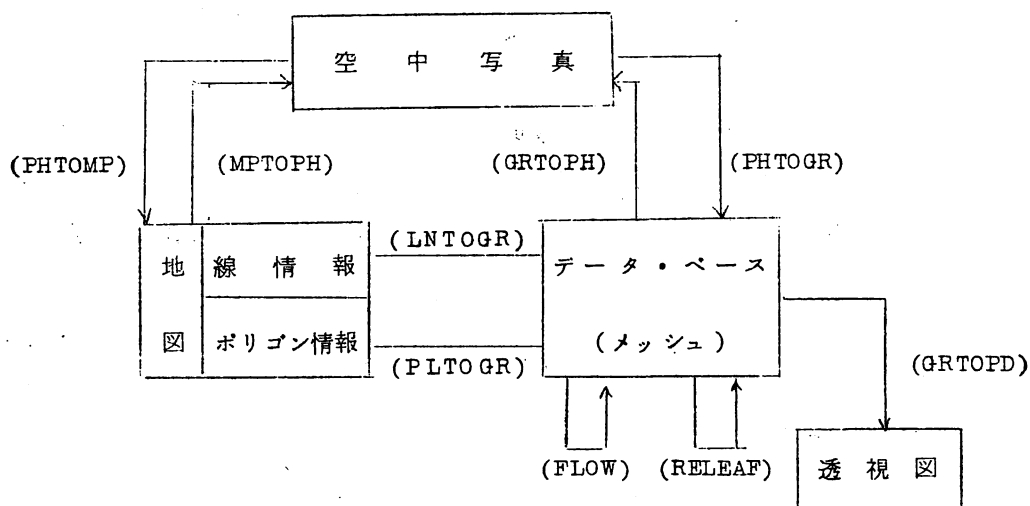
図-2 各種情報のオーバーレイ用ソフトウェアシステム
