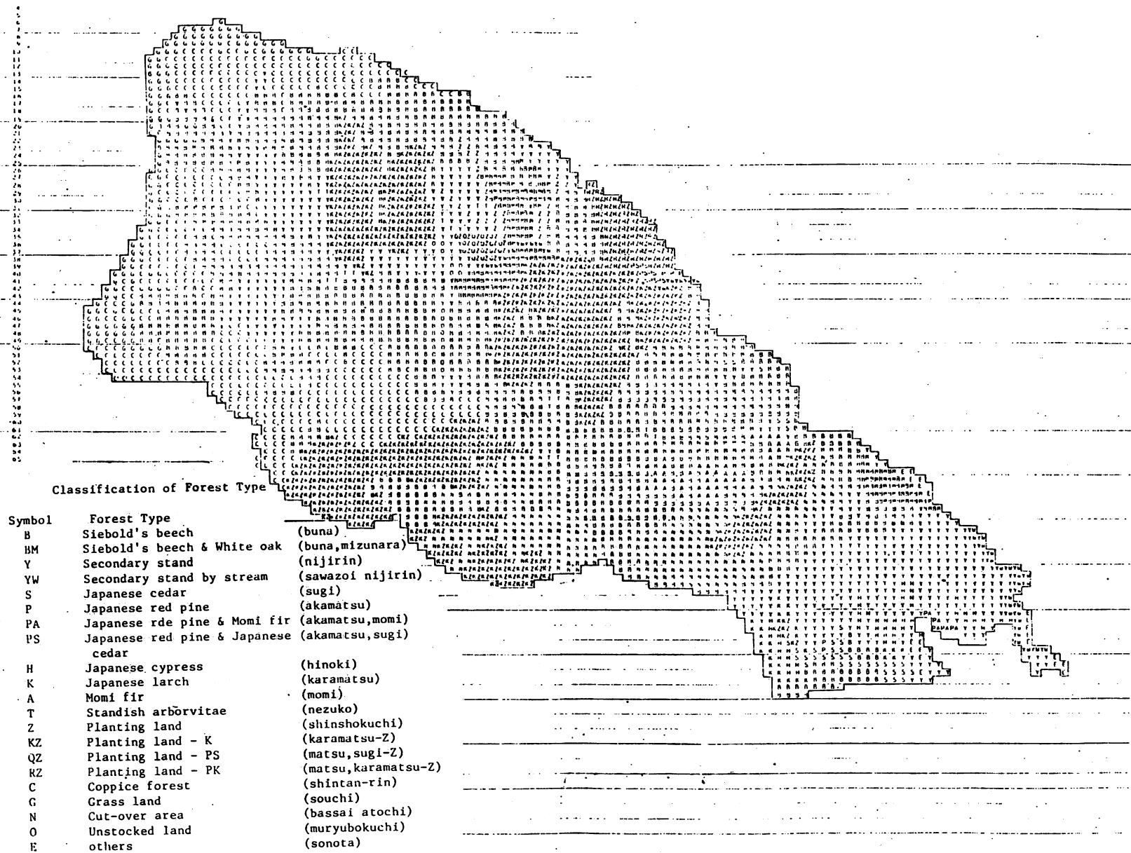
図9 樹種区分図
