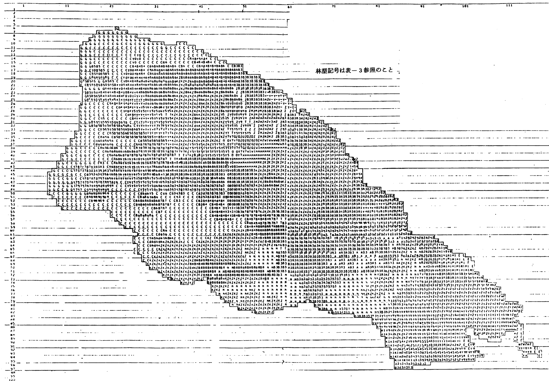
図8 林型区分図
