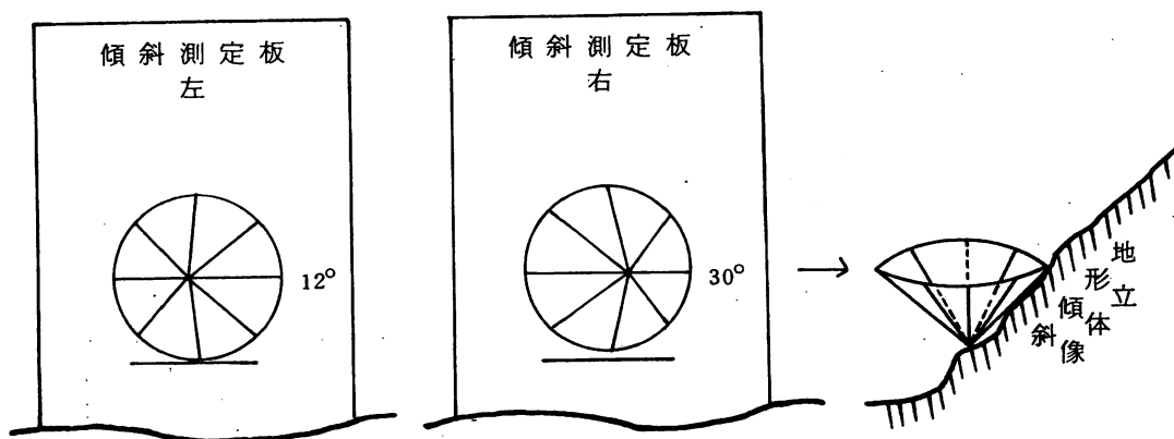
図一 1 1 傾斜測定板による傾斜角の測定
