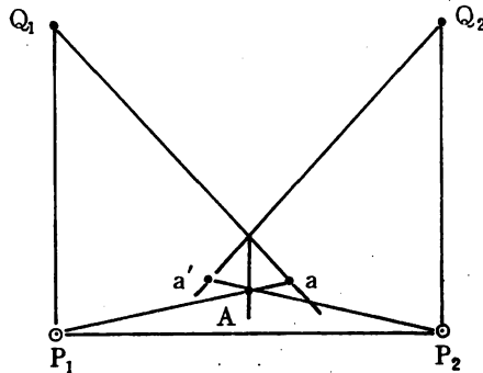
図一 1 4 写真基線附近の交会法
