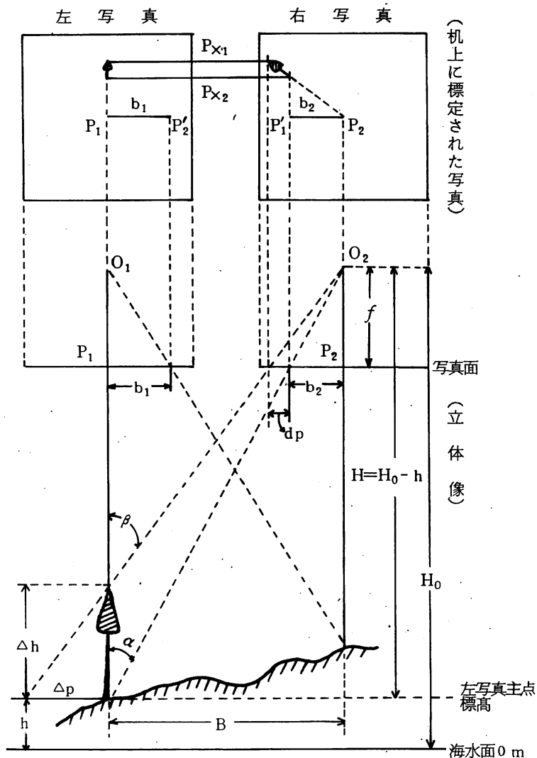
図一7 地物の標高測定
