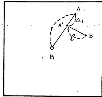
図-10 2点間の水平距離の求め方
