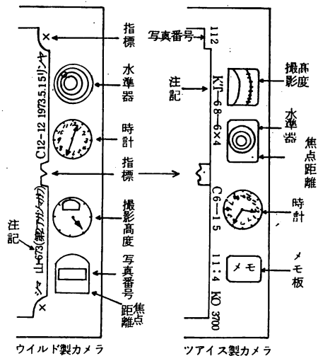
図-1 写真の計器と注記
