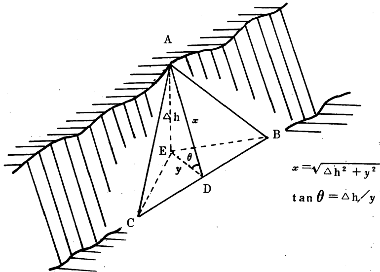
図—1 2 崖の高さと斜面長の測定
