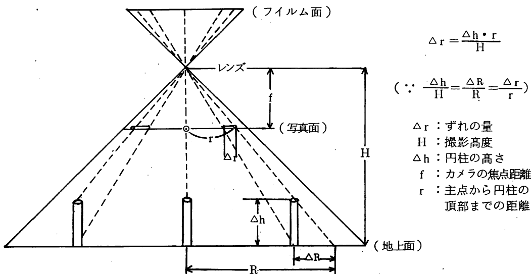
図-2 B 中心投影による画像のずれ
