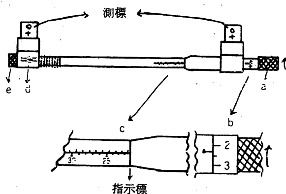
図一八 視差測定棒
