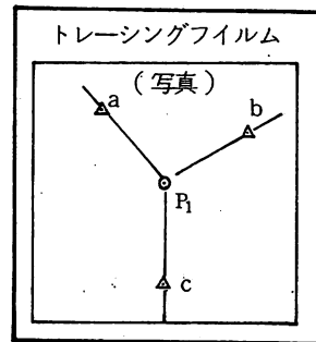
図一 9 主点を地図へ移写する方法
