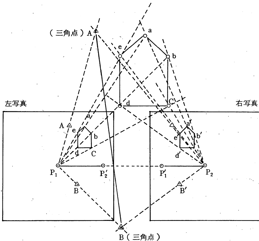
図-13 交会法による図化
