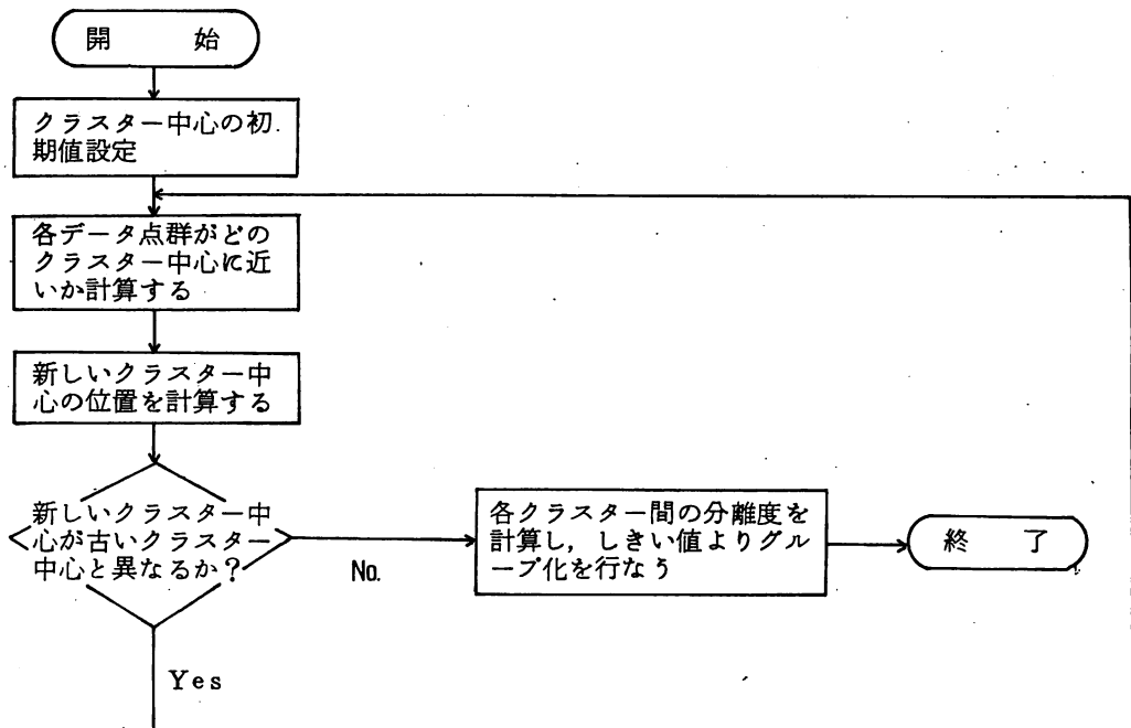
図 3 - 1 クラスタリング・アルゴリズム
