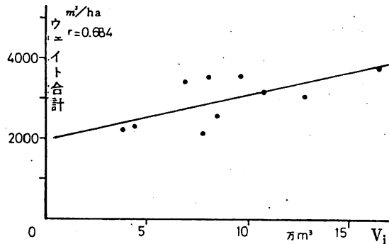
図 5-5 P S U 推定材積とウェイト合計
