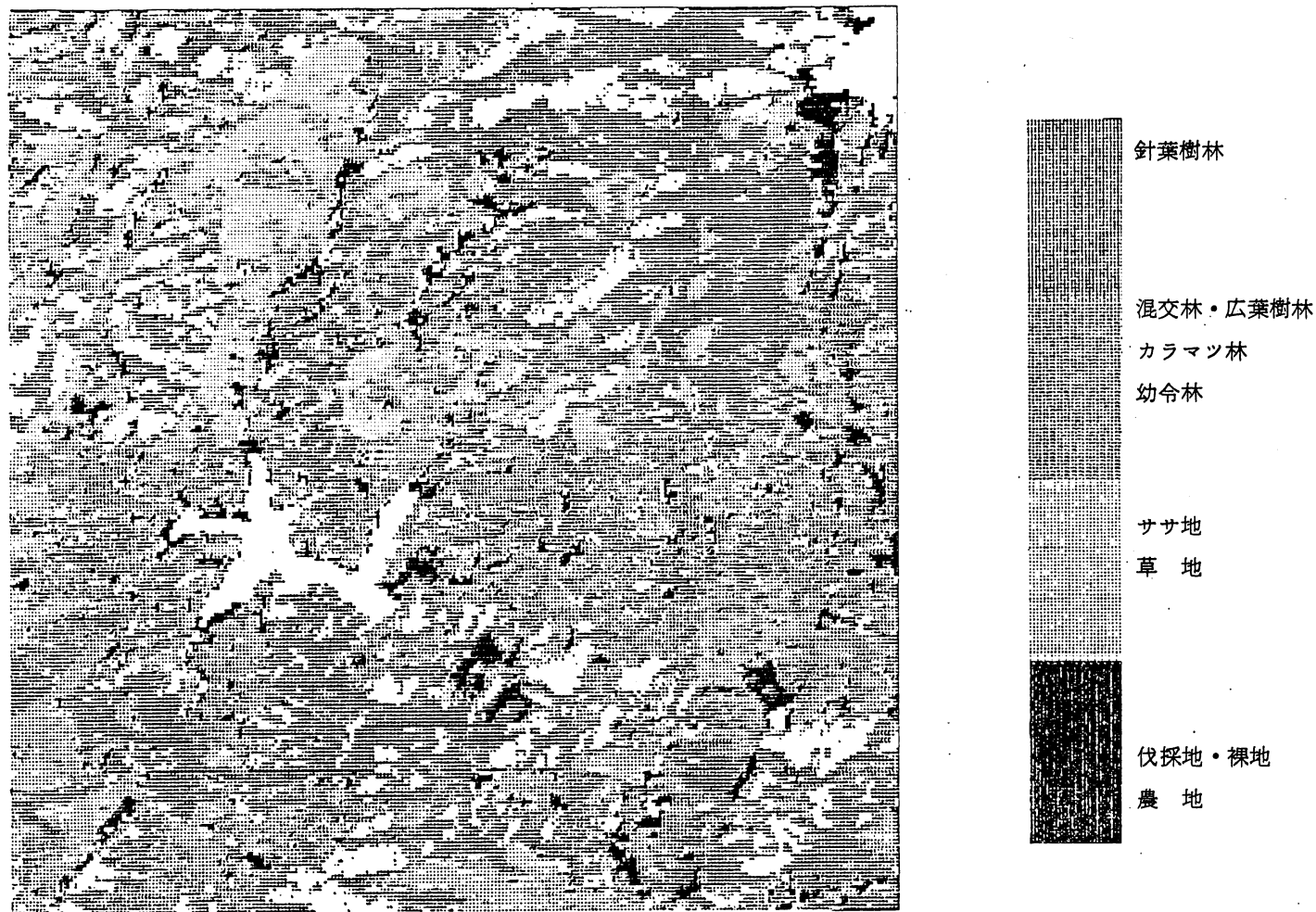
図 3-3 2 時期 8 次元ランドサットデータによる森林被覆タイプ区分結果を X-Y プロッターで図面化したもの
