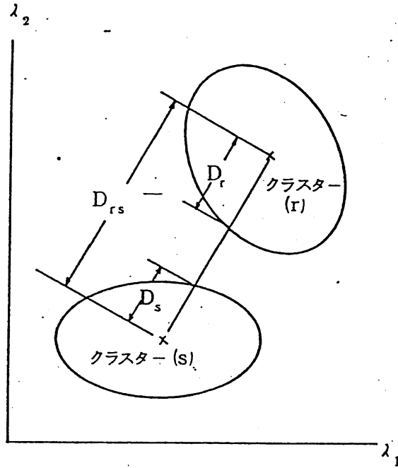
図 8-2 クラスタ間の分離度
