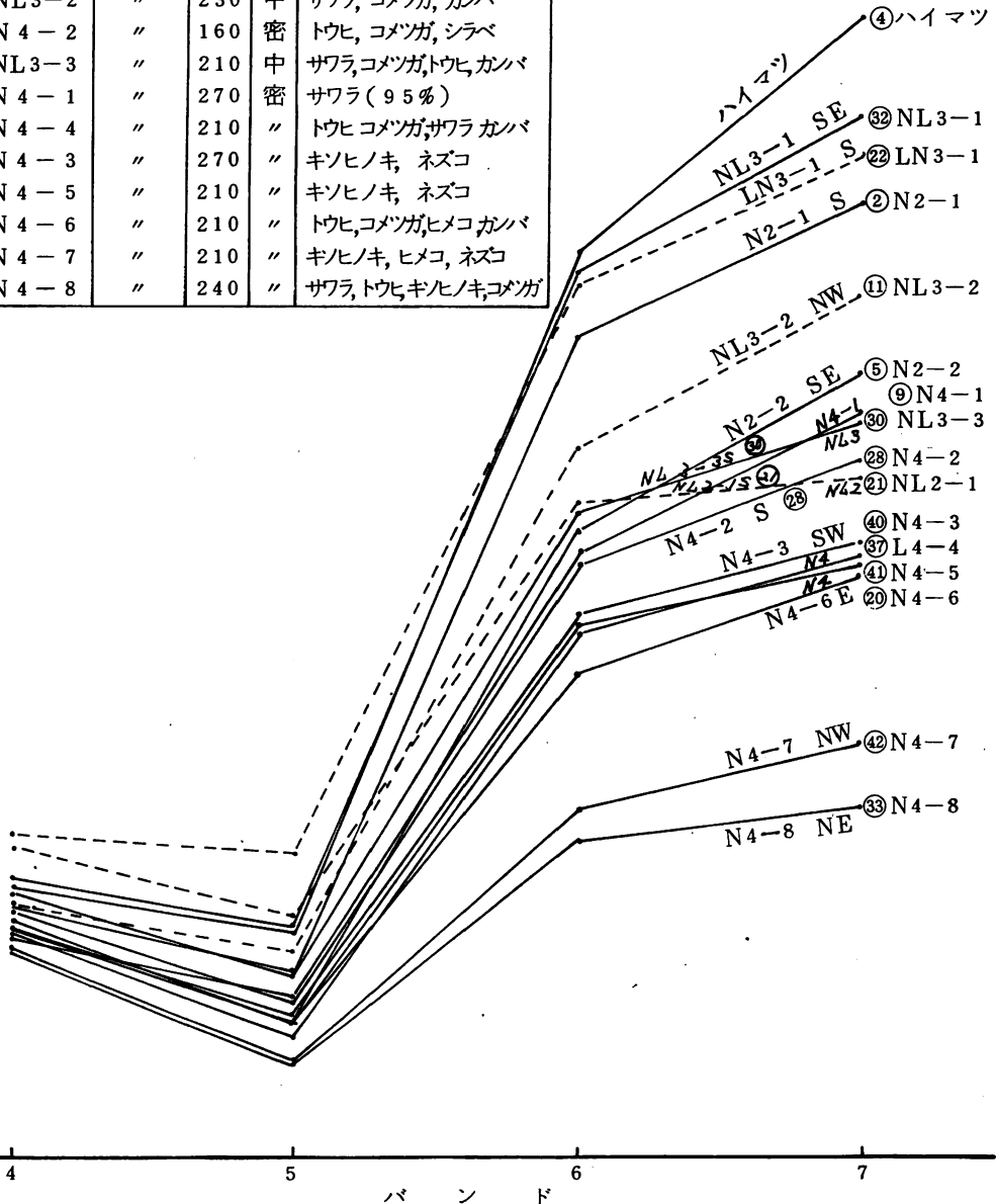
図2-1 (1) トレーニングエリアのランドサットデータの特徴
