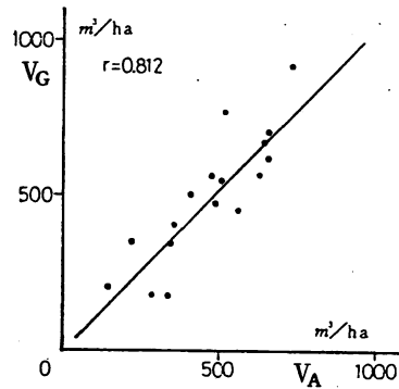
図 5-4 判読材積と現地調査材積
