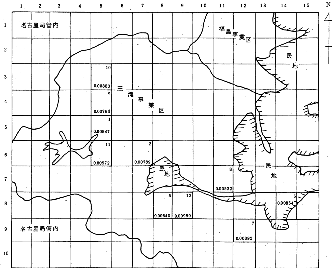
図 5 - 2 抽出された第 1 次抽出プロット (PSII) の配置図とその抽出確率 (ni)
