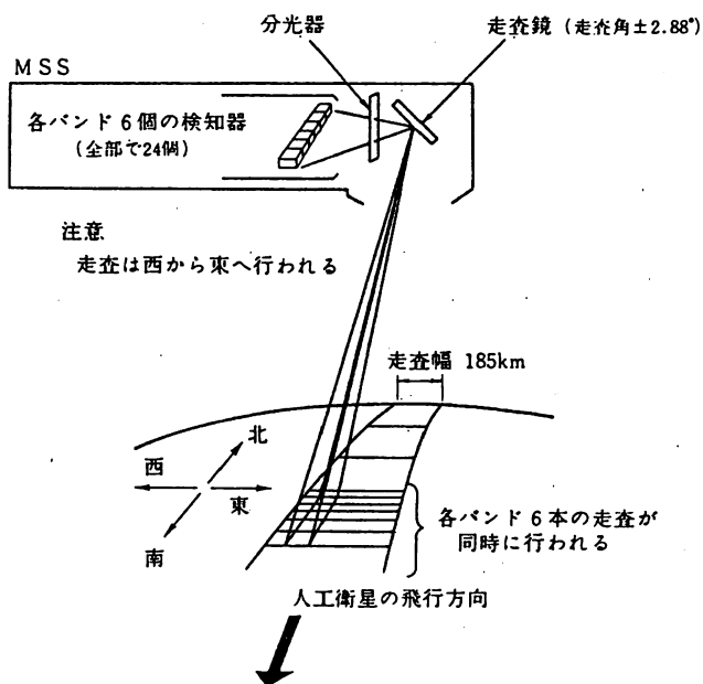
図 1-1 ランドサットのMSSによる観測
