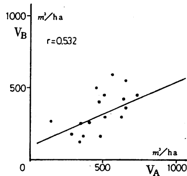
図 5-7 判読材積と調査簿記載値
