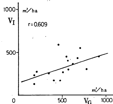
図 5-6 現地調査材積と調査簿記載値
