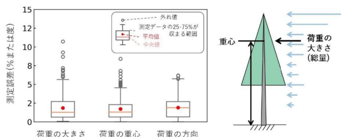
図2 荷重の計測精度
