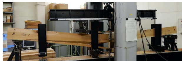
図1 コウヨウザンの曲げ強度試験の様子
