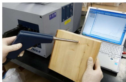
図2 近赤外分光法による非破壊での木材の樹種識別 光が出るプローブの先端を木材の表面に軽く当てて測定します。
