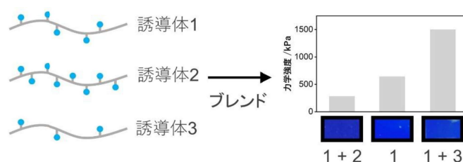
図2 セルロース誘導体のブレンドによる色相と力学物性の独立制御
