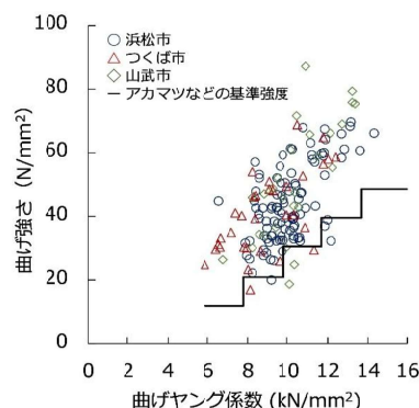
図2 コウヨウザンの曲げヤング係数(たわみにくさ)と曲げ強さとの関係
