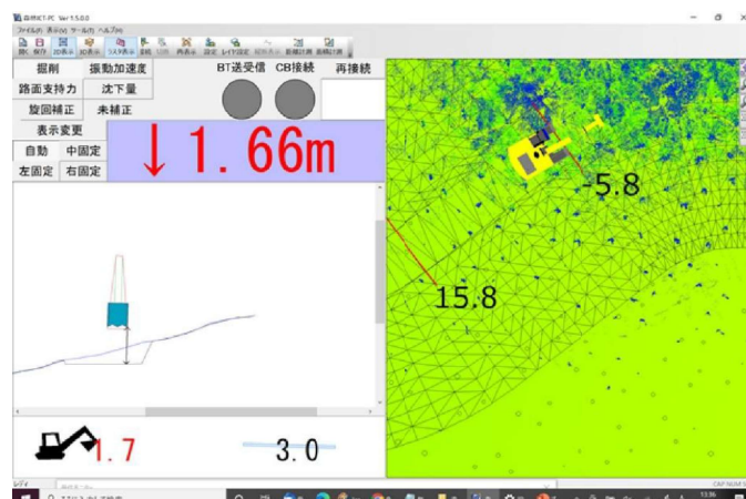
図1 ガイダンスモニター
