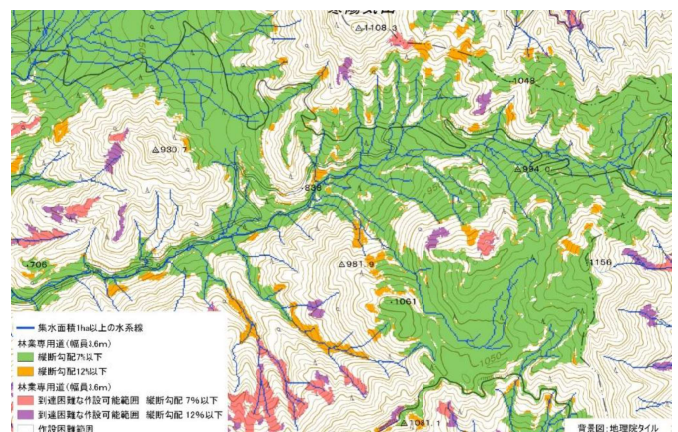
図1 路網整備難易度推定図
