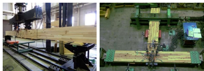
図2 間柱を用いて製造した大断面集成材の強度試験 (左:曲げ強度試験、右:接合性能試験)
