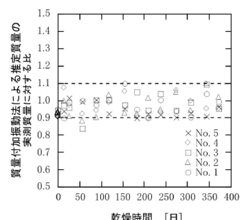
図2 質量付加振動法による棧積み平角の推定結果 (Kubojima et al. 2024を一部改変) 質量付加振動法によって、棧積み状態の平角の重さをほとんどの場合で実測値の±10%の範囲で推定できました。
