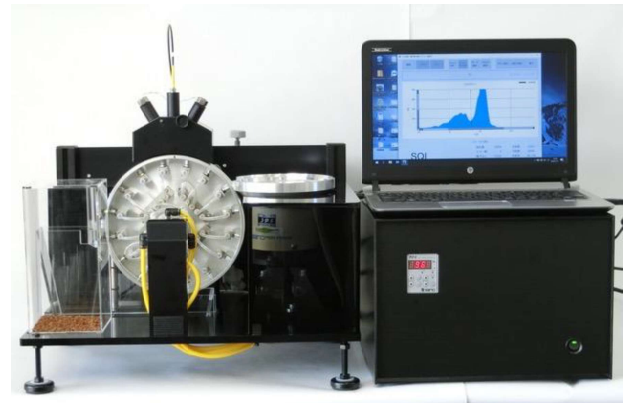
図1 充実種子選別装置
