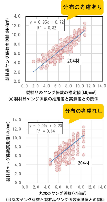
図1 丸太段階で製材品のヤング係数を評価する 様々な木取りが適用でき一度に多くの製材品を生産できる大径材の場合には、ヤング係数の丸太内部の「分布」を考慮することで製材品ヤング係数の推定精度が高くなります。
