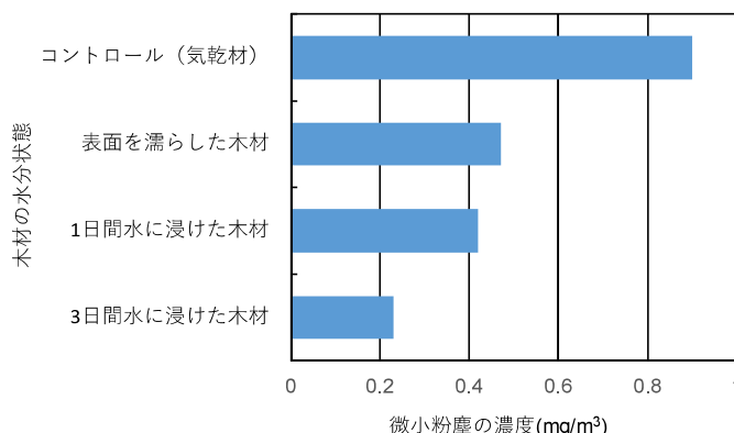
図1 丸鋸切削時に発生する微小粉塵の質量濃度 木材の切削前に水分を付与することで丸鋸切削時に発生する粉塵を半分に以下にできることを明らかにしました。
