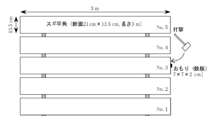
図1 天然乾燥過程におけるスズ棧積み平角の重さの推定 (Kubojima et al. 2024を一部改変) 天然乾燥過程において、おもりのない状態と付着した状態でスズ平角の木口面を打撃し、打撃音の高さを測定しました。
