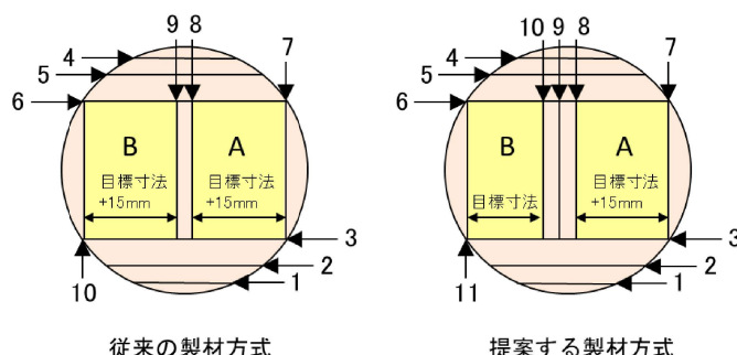
図2 スギ大径材の製材方式
