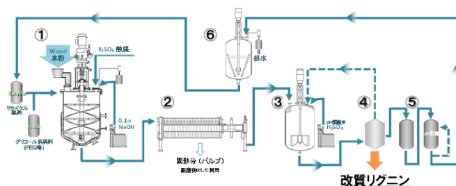
図1 改質リグニン製造プロセスの概要
