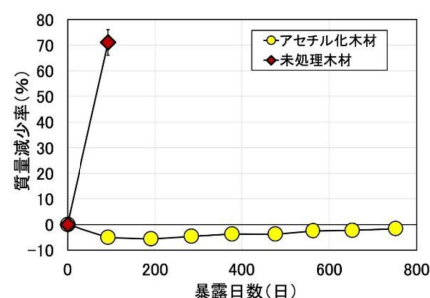
図2 海中暴露試験によるアセチル化木材と未処理木材の質量減少率の変化
