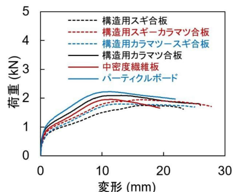
図1 くぎのせん断性能を調べる試験の様子と試験結果の一例 日本ツーバイフォー建築協会が定める接合部の試験を実施し、荷重と変形の関係測定しました。この試験結果から力学的特性値を明らかにしました。
