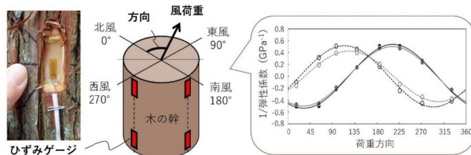
図1 風荷重の計測イメージ
