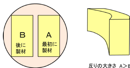
図1 心去り平角の製材順と反りの関係
