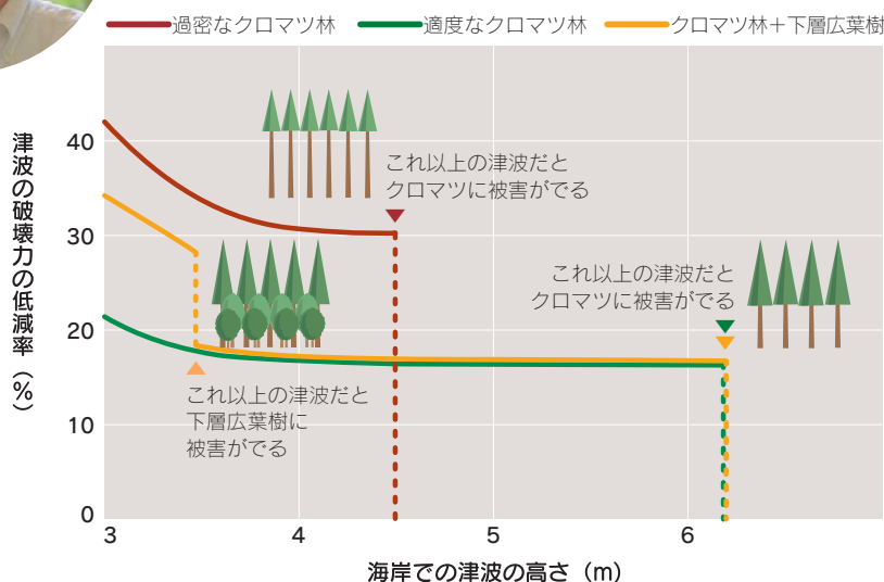
図1 林型による津波の破壊力の低減率と林帯の耐性の違い (林帯幅 200 m の例)
